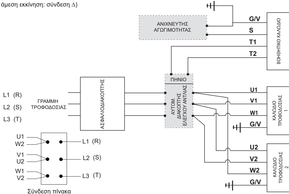
Καλώδιο τροφοδοσίας 1
