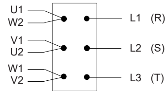
Conexión cuadro
