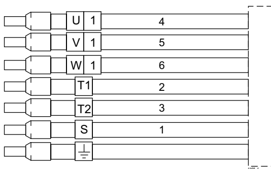
Schalttafelanschluss
