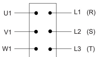
Branchement tableau
