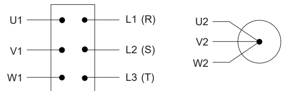
Σύνδεση πίνακα
