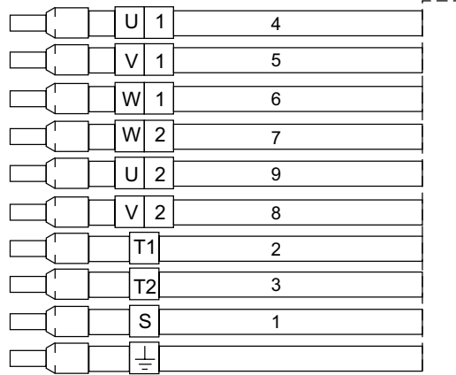
Σύνδεση πίνακα
