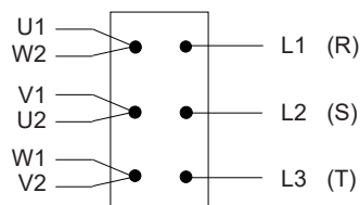
Branchement tableau
